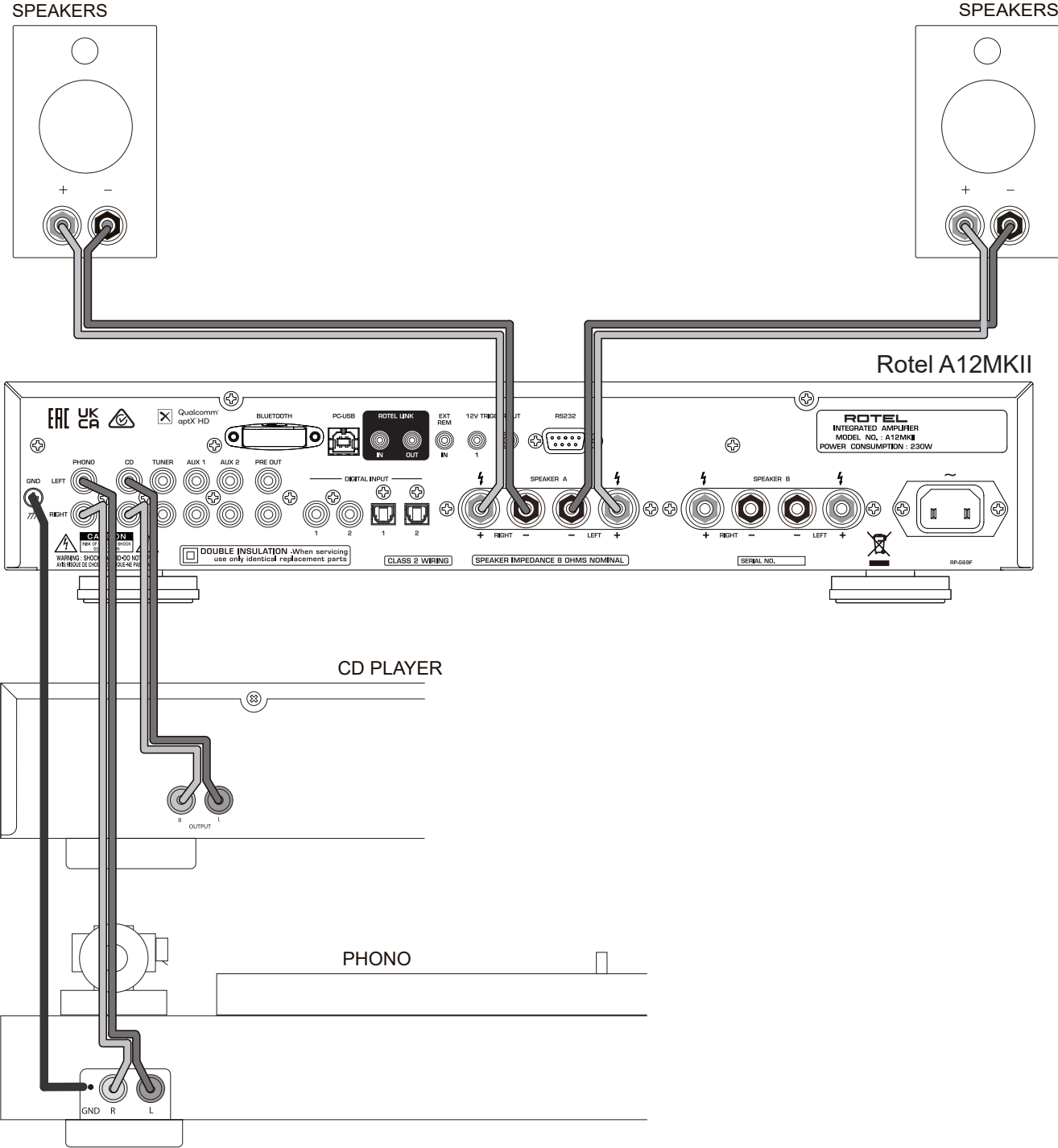
Figure 3: Preamp Input and Speaker Output Connections Branchements des entrées sources et sorties enceintes acoustiques Anschlussdiagramm Conexiones para Entrada de Señal y Salida a las Cajas Acústicas Collegamenti ingressi e diffusori De signaalgangen en de luidsprekeruitgangen Signal- och högtalaranslutningar Подсоединение источников сигнала и акустических систем
